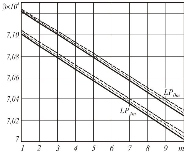
Рис. 14. Распределение значений \beta высших мод LP_{lm} по радиальному порядку m
