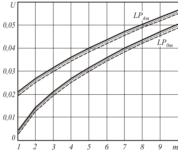
Рис. 13. Распределение значений U высших мод LP_{lm} по радиальному порядку m
