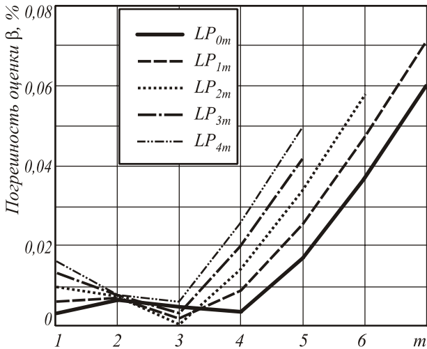
Рис. 8. Распределение значений погрешности оценки \beta высших мод LP_{lm} по радиальному порядку m
