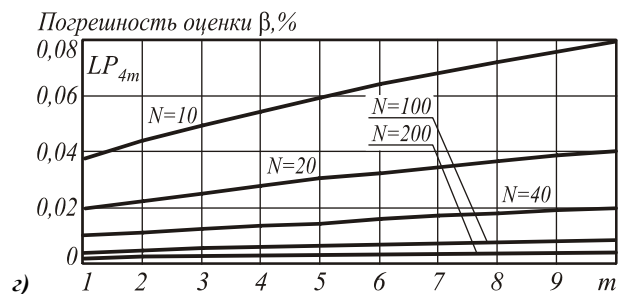
Рис. 15. Распределение значений погрешности оценки параметров передачи высших мод LP_{lm} по радиальному порядку m
