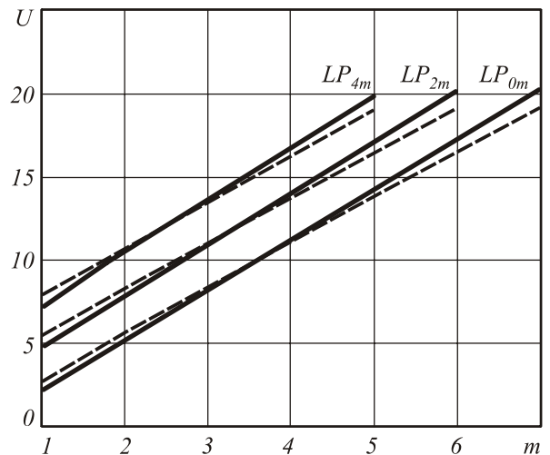
Рис. 5. Распределение значений U высших мод LP_{lm} по радиальному порядку t
