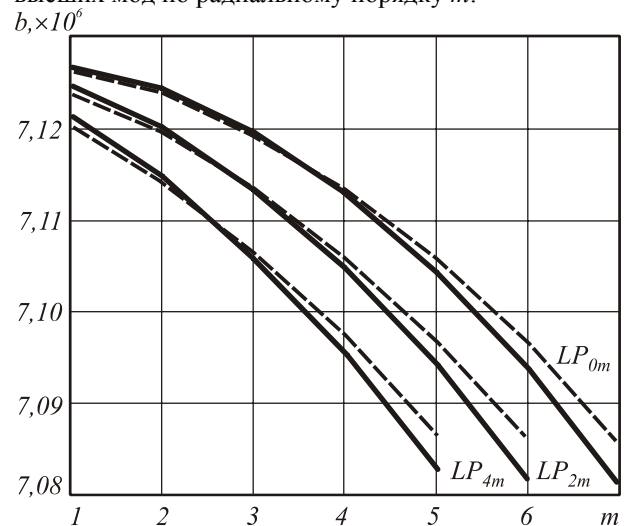
Рис. 6. Распределение значений \beta высших мод LP_{lm} по радиальному порядку t
