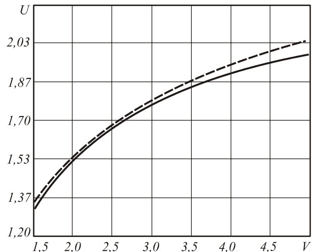
Рис. 2. Зависимость параметра моды в сердцевине U от нормированной частоты V
