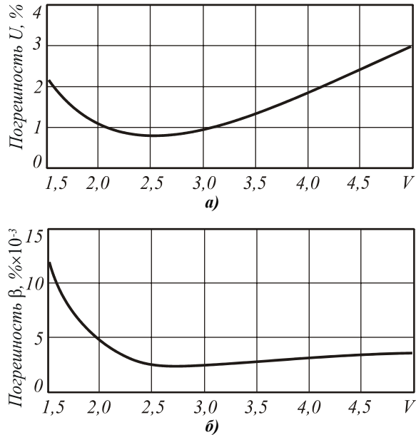
Рис. 4. Погрешность предложенного метода: а) параметр моды в сердцевине U ; б) постоянная распространения \beta
