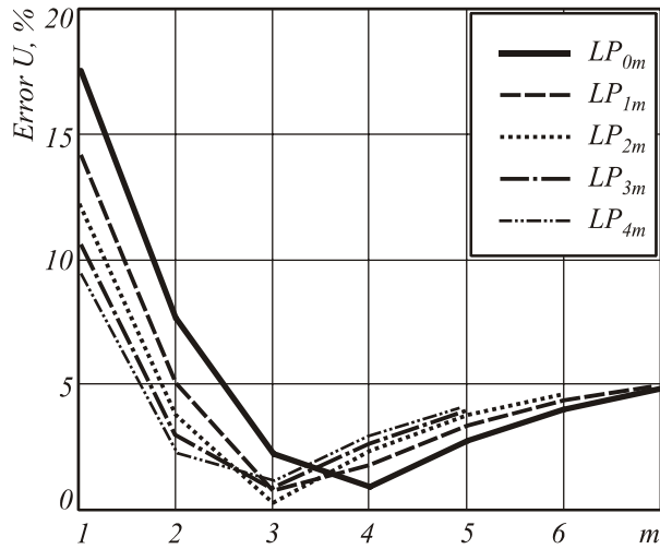
Рис. 7. Распределение значений погрешности оценки U высших мод LP_{lm} по радиальному порядку m
