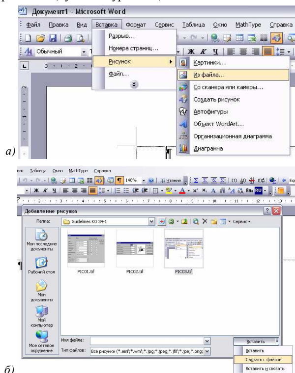
Рис. 2. Линковка рисунков
