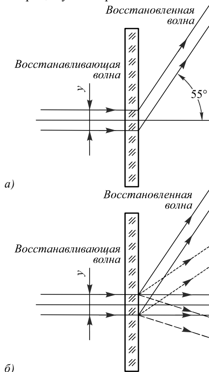
Рис. 6. Схемы дифракции лазерного излучения на одиночной ячейке матрицы объёмных субголограмм, где а) отклонение пучка лазерного излучения на одной длине волны в 1-й порядок дифракции; б) отклонение трёх пучков лазерного излучения на трёх длинах волн также в 1-й порядок дифракции
