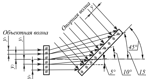
Рис. 5. Запись голограммы. Для записи используется технологическая матрица голограмм, отклоняющая пучки на 0^\circ , 5^\circ , 10^\circ и 15^\circ соответственно. Для снижения требований к технологической голограмме заготовка повернута на 45^\circ
