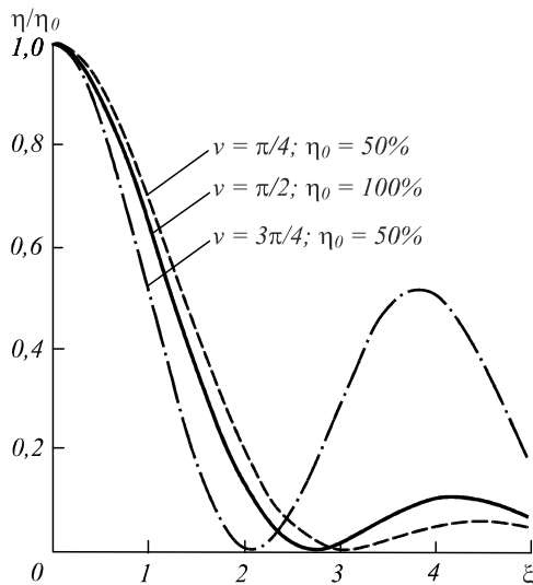
Рис. 4. Зависимость относительной дифракционной эффективности \eta/\eta_0 пропускающей объёмной субголограммы от параметра \zeta = \delta(2\pi/\lambda)T \sin \theta_0 для различных значений параметра \nu = \pi n_1 T / \lambda \cos \theta_0
