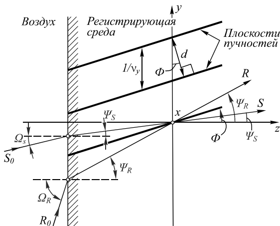
Рис. 1. Образование объёмной голограммы.
