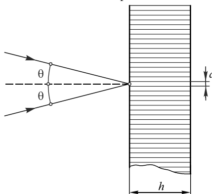
Рис. 2. Схема записи объёмной голограммы. Вследствие интерференции двух пучков света в среде образуются плоскости пучностей, \theta – угол между лучом и нормалью к поверхности, h – толщина фотоносителя, d – период голограммы
