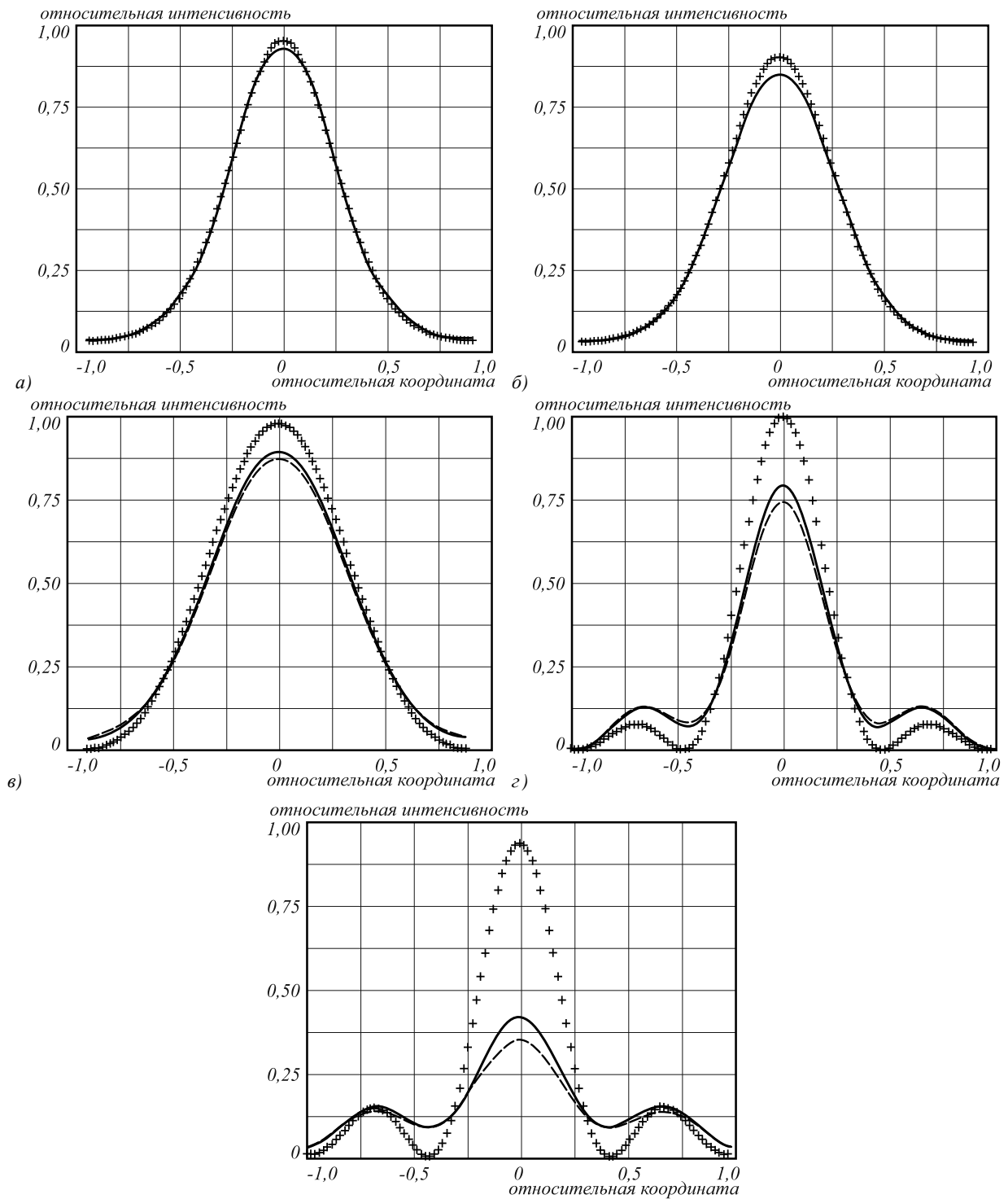
Рис. 1. Распределение интенсивности в фокальной плоскости дифракционной линзы z = f : f = 200\lambda (а); f = 100\lambda (б); f = 50\lambda (в); f = 20\lambda (г); u z = 1,5f, f = 20\lambda (д)
