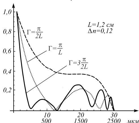
Рис. 1. Зависимость кривой видности от величины расстройки \Delta при разных значениях мощности звуковой волны для любого положения окна прозрачности АОФ, при условии, что в пределах основного спектрального диапазона АОФ изменение спектрального распределения светового пучка незначительно
