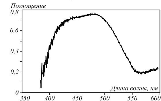
Рис. 1. Спектр поглощения тонкой плёнки азополимера. Толщина плёнки 1600 нм
