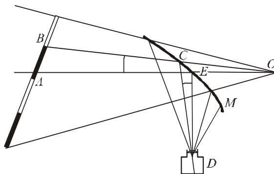
Рис. 6. Схема расположения зеркала между предметом и камерой
