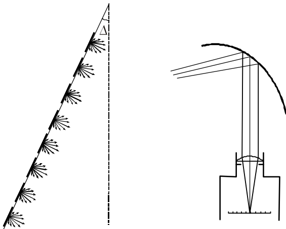
Рис. 7. Взаимное расположение предмета, зеркала и камеры для проверки свойств зеркала методом трассировки лучей
