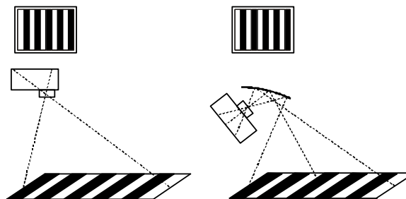
Рис. 2. Исправление перспективных искажений
