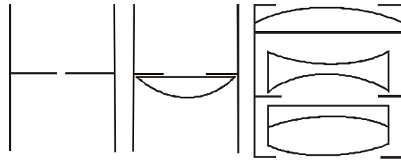
Рис. 8. Различные объективы, использованные для получения изображения методом трассировки лучей
