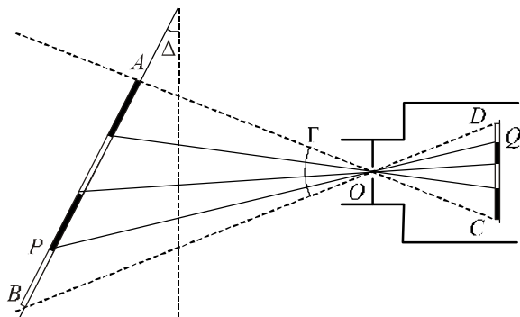
Рис. 3. Формирование изображения предмета, расположенного под углом к плоскости изображения
