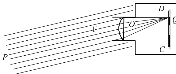
Рис. 5. Предмет расположен на значительном удалении от камеры
